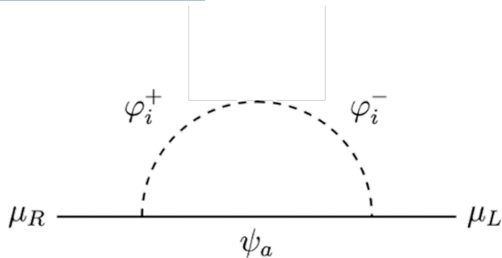
Muon mass
