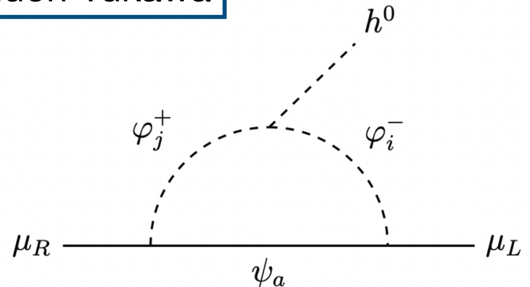
Muon Yukawa
